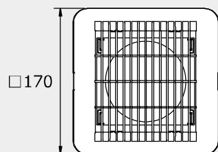
フロントパネル外形寸法
