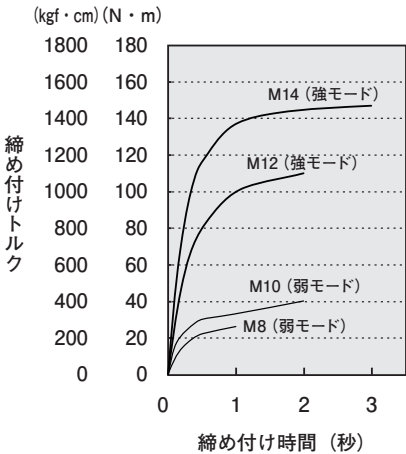
普通ボルト
