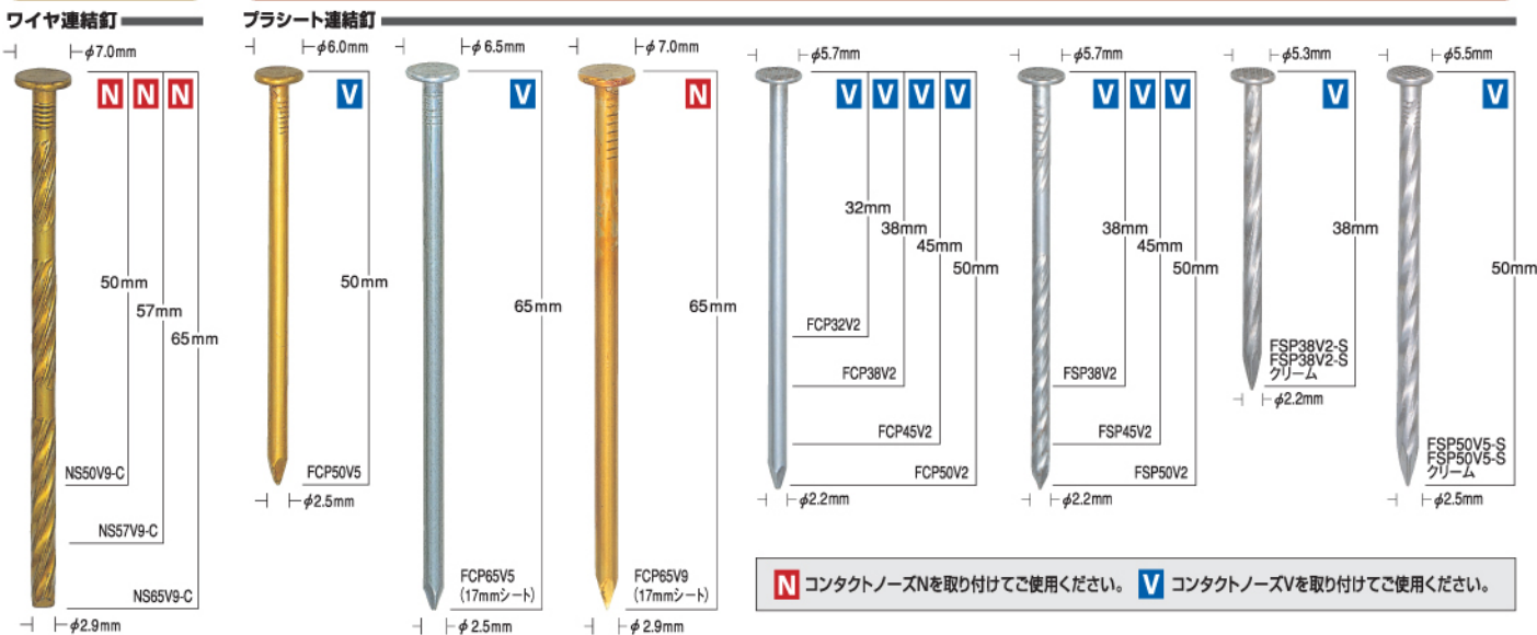
HN-65N1 使用釘
