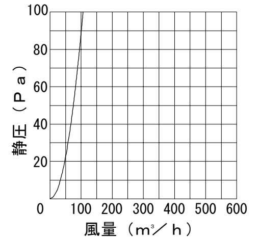
圧力損失曲線
