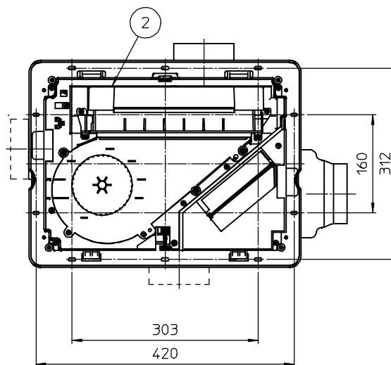
取付寸法図 (補強材)
