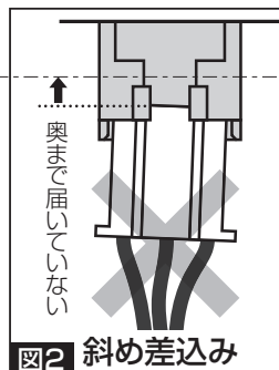
図2 斜め差込み
