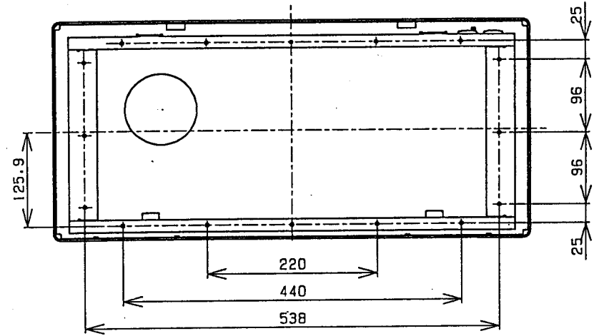
(裏面図)
