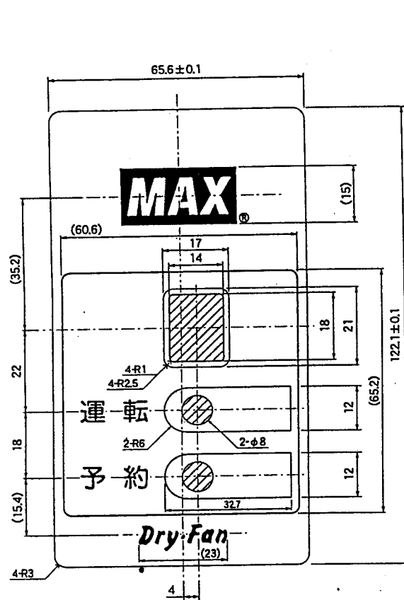
一般寸法図
