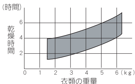
衣類の重量と乾燥時間 浴室周辺温度：20℃ 浴室周辺湿度：60%
