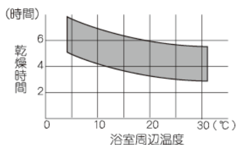
浴室周辺温度の変化と乾燥時間
