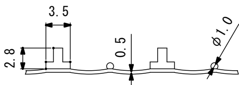
断面詳細図
