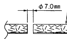
アンカー下穴詳細図
