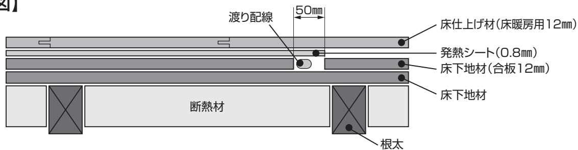
【準防火納まり図】(石膏ボードを使用する場合)
