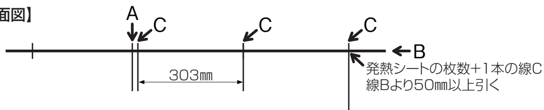
【平面図】
