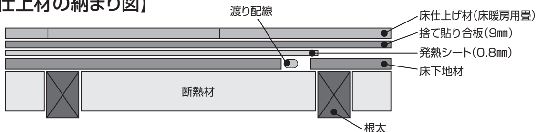
【床暖房用畳仕上材の納まり図】
