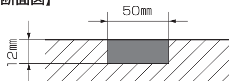
【断面図】
