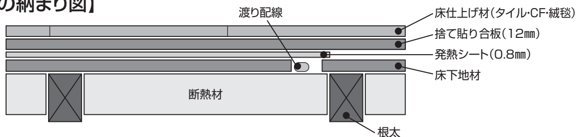
【軟質仕上材の納まり図】
