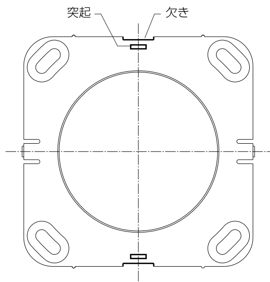
副吸込グリルジョイントの向き…突起が縦側
