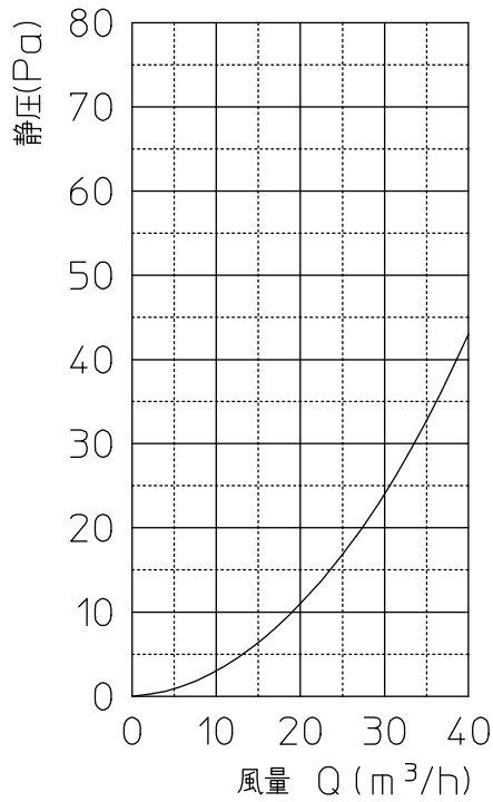
○圧損特性曲線
