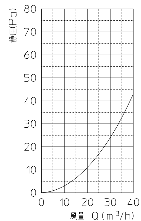
○圧損特性曲線
