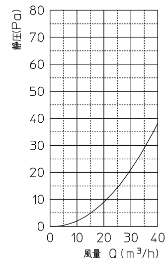
○圧損特性曲線
