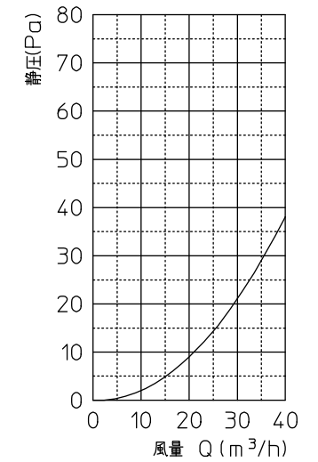
○圧損特性曲線
