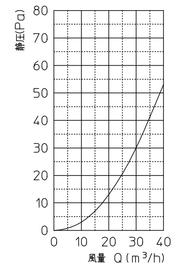
○圧損特性曲線
