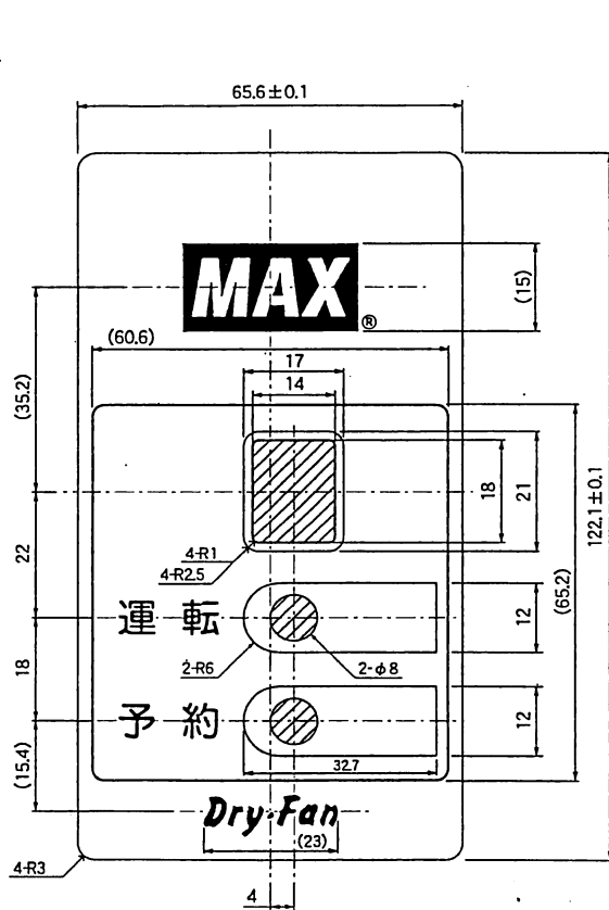
一般寸法図
