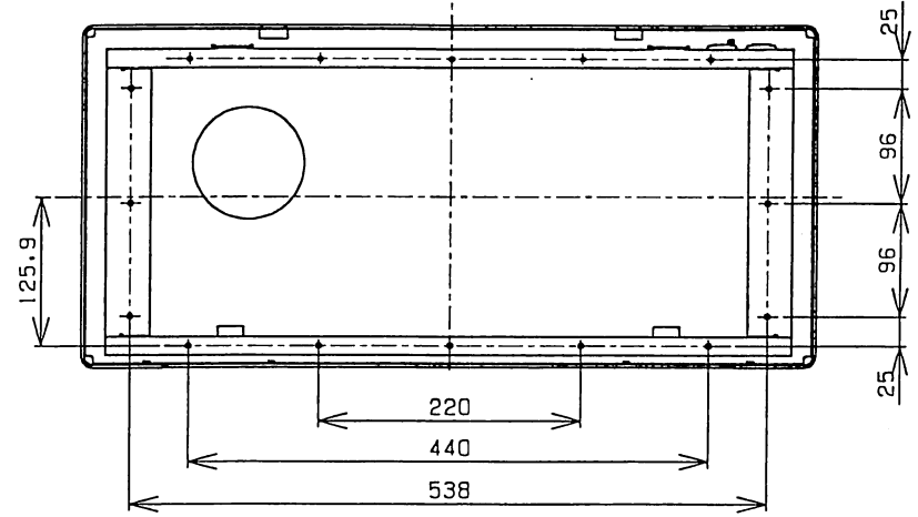
(裏面図)
