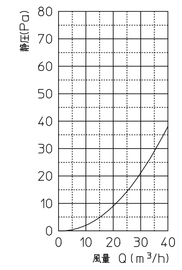
○圧損特性曲線
