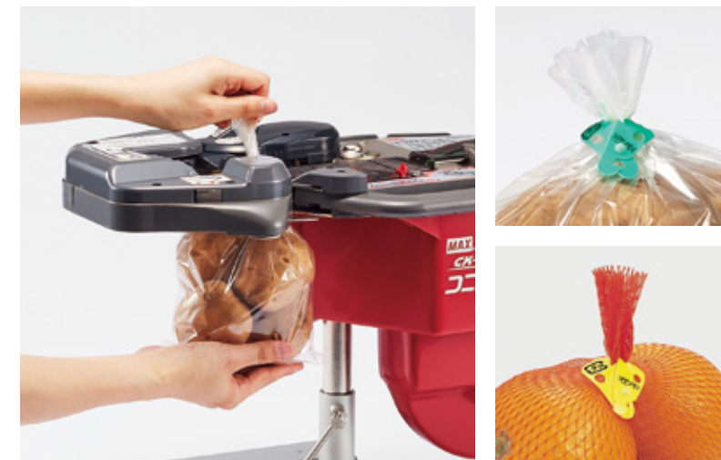
包装作業の効率化を実現する青果・食品用袋口結束機「コニクリッパ」と簡単開封が可能な専用結束具「コニクリップ」
