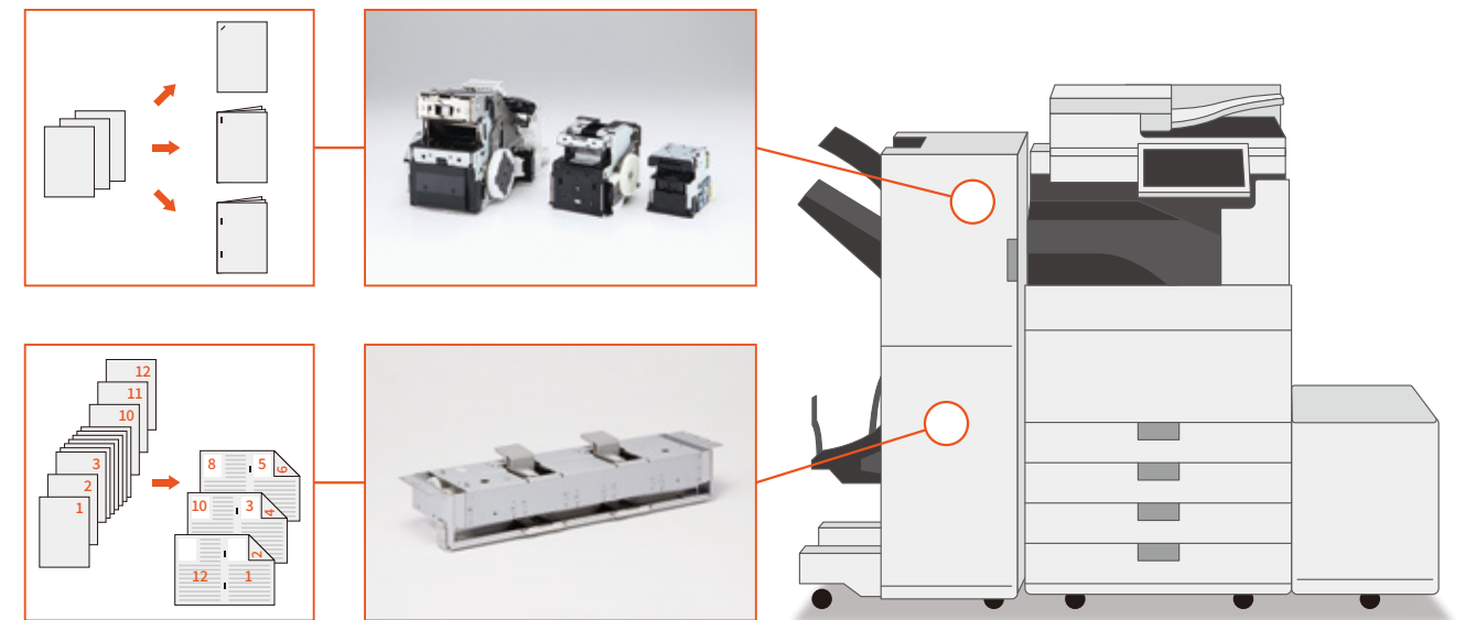
簡易製本市場向けの「中とし用オートステープラ」
