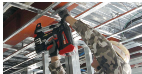
コードレス ガス内燃式ピン打機「ガスネイラ」
