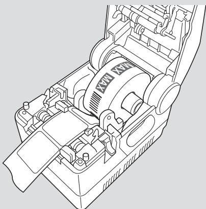
(剥離ユニットからラベル紙を外してセットした状態)
