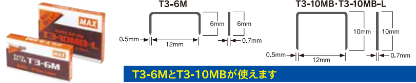
TH-V2 使用ステープル実寸図 (線径：幅0.7mm×厚さ：0.5mm)
