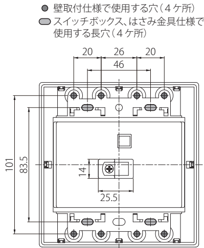
裏面図
