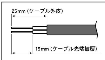
ケーブル被覆のむき寸法
